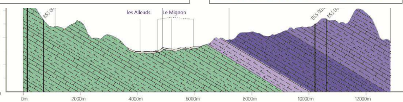
Coupes interprétatives Terraqua
